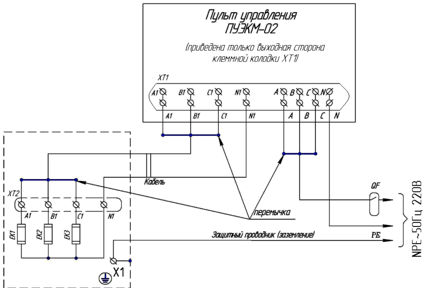
Рисунок 4 – схема подключения электрокаменок ЭКМ-1-4,5 и ЭКМ-1-6 к однофазной сети ~50Гц/220В при питании от пульта ПУЭКМ-02
